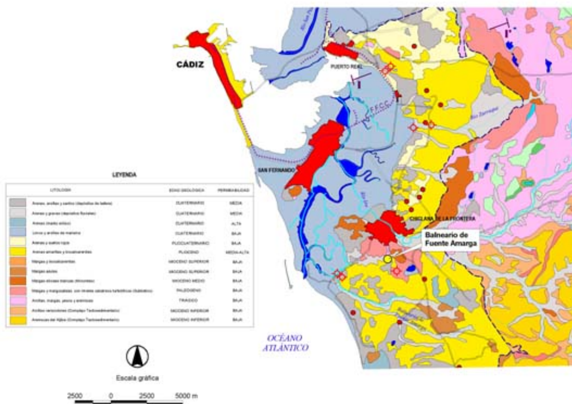
Esquema hidrogeológico (Lugares de Interés Geológico de Andalucía, IGME)
