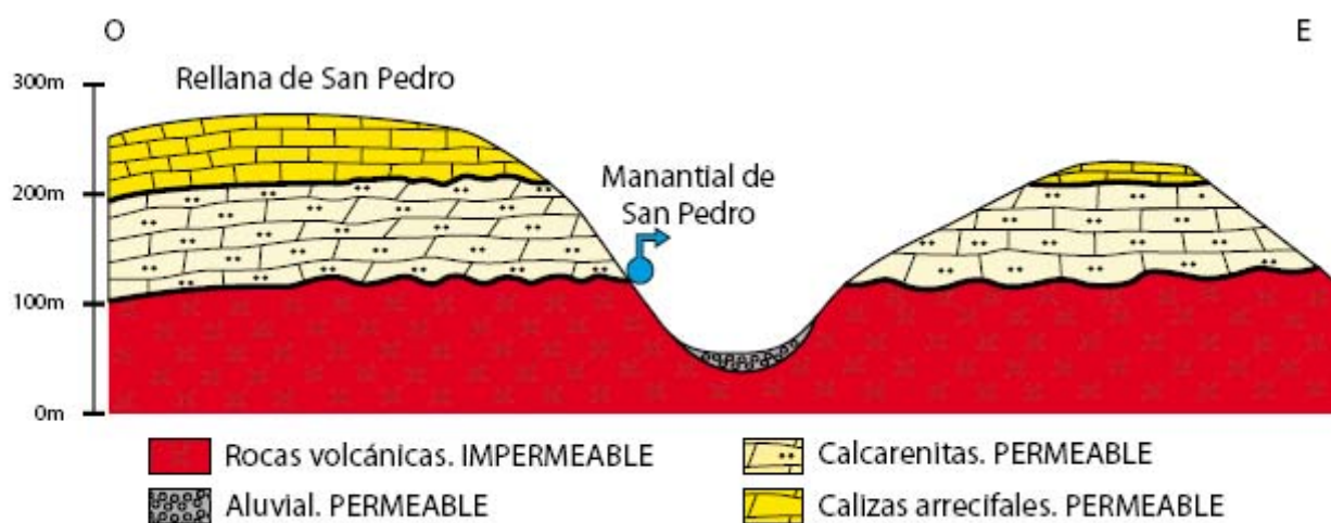
Corte hidrogeológico (IGME,(2010)
