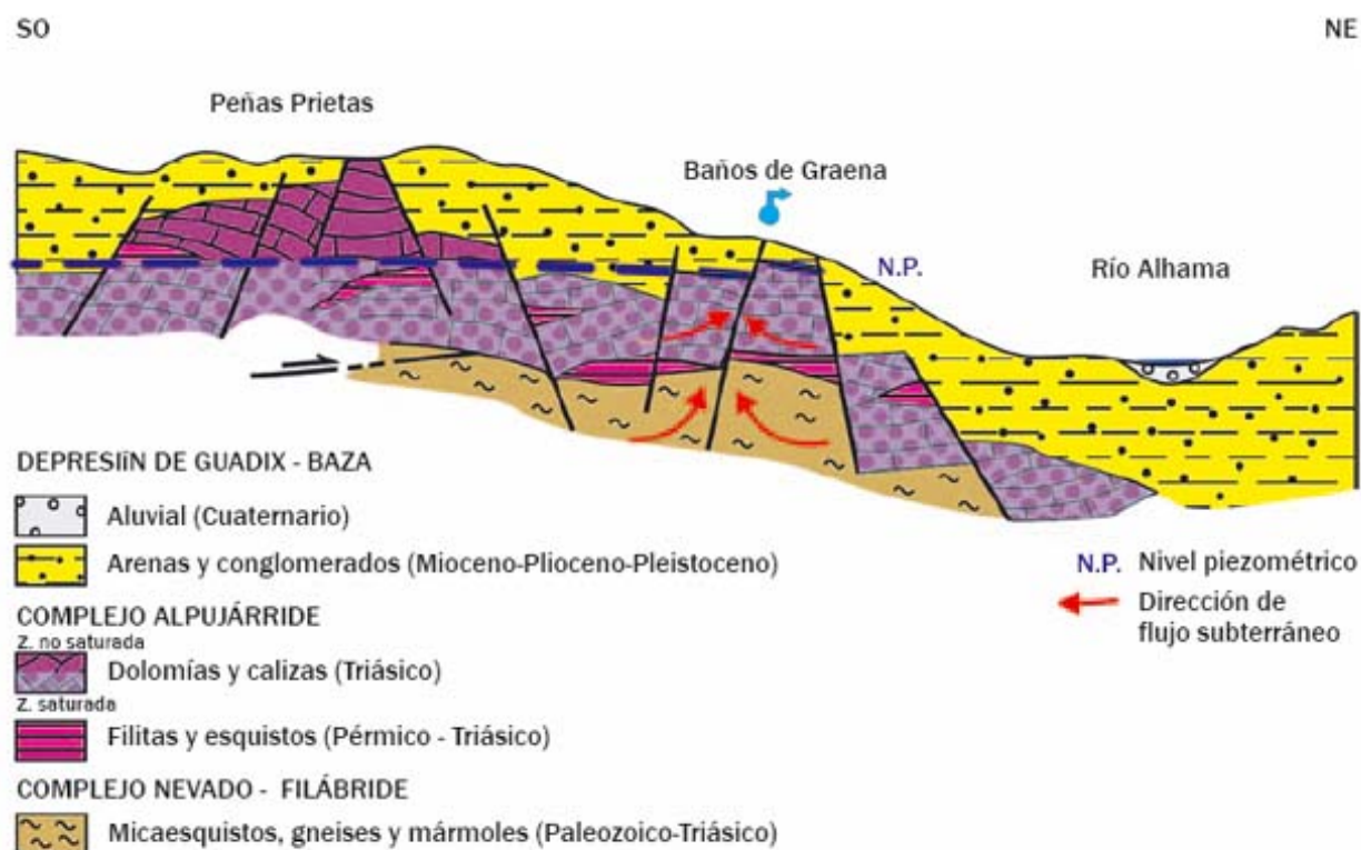
✦ CORTE HIDROGEOLÓGICO DE LOS BAÑOS DE GRAENA
