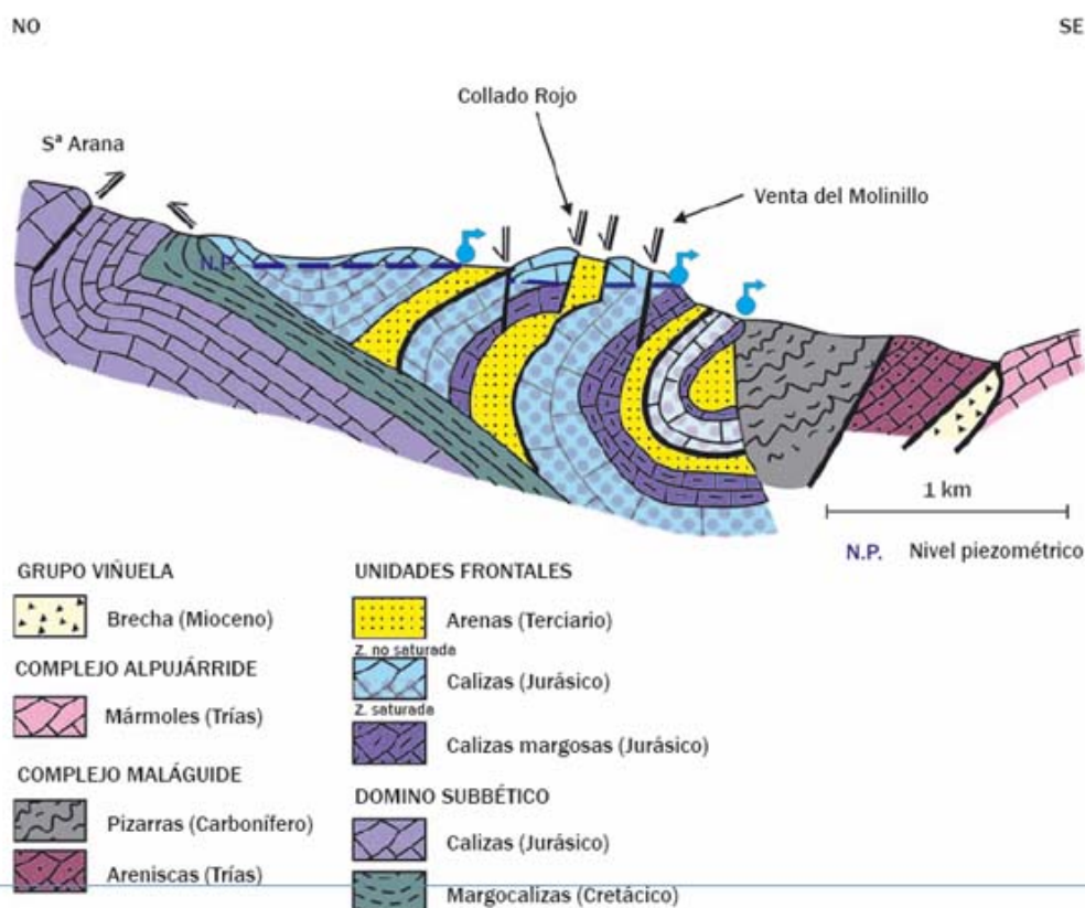
✦ CORTE HIDROGEOLÓGICO DE LA CABECERA DEL RÍO FARDES
