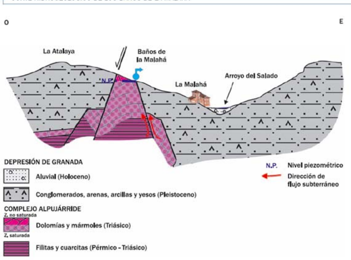
✦ CORTE HIDROGEOLÓGICO DE LOS BAÑOS DE LA MALAHÁ
