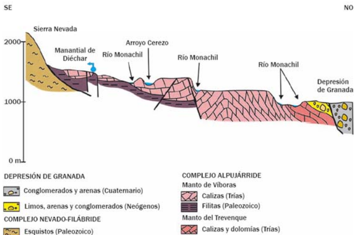
✦ CORTE HIDROGEOLÓGICO DEL MANANTIAL DE DIÉCHAR Y RÍO MONACHIL
