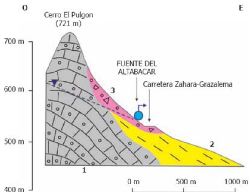
Esquema hidrogeológico de la fuente del Altabacar
