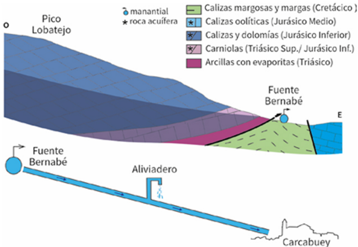
Corte geológico de la Fuente de Bernabé (Fuentes y manantiales de las Sierras Subbéticas, Felipe González Barrionuevo, 2025)
