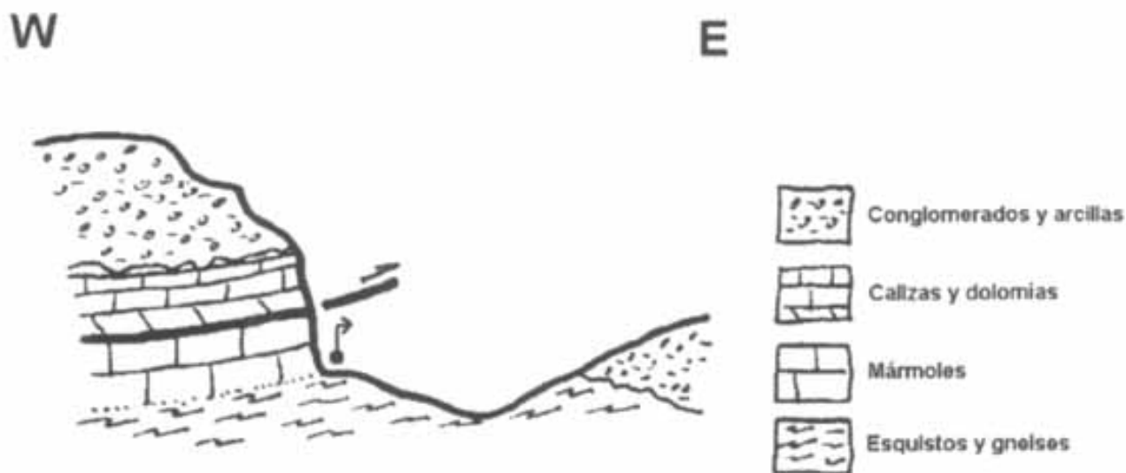
Esquema hidrogeológico (Atlas Hidrogeológico de la Provincia de Granada. (Diputación de Granada – IGME 1988)
