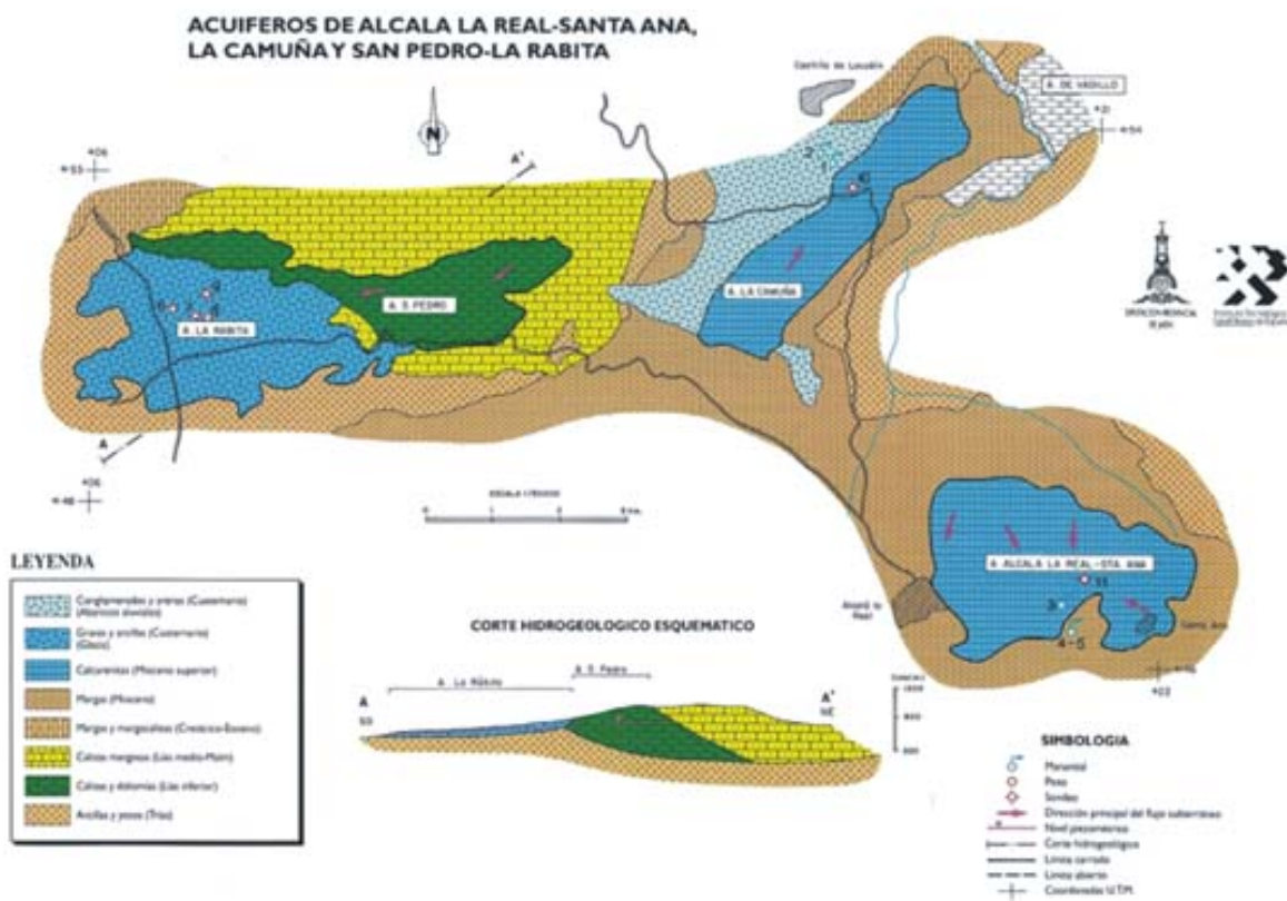
Esquema y corte hidrogeológico (IGME Granada)
