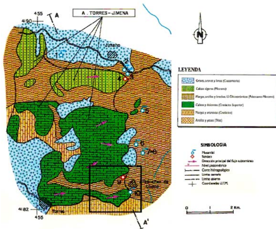
Esquema hidrogeológico (IGME Ganada)
