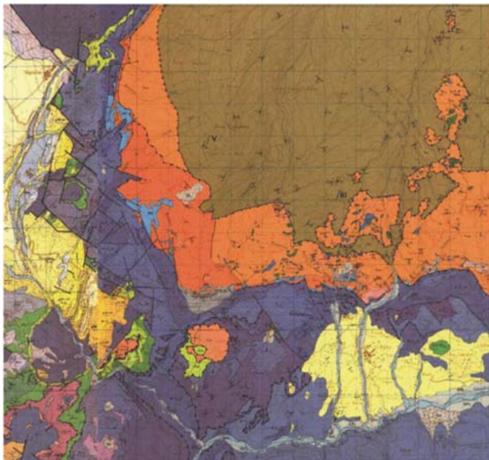
Esquema hidrogeológico (IGME Granada)
