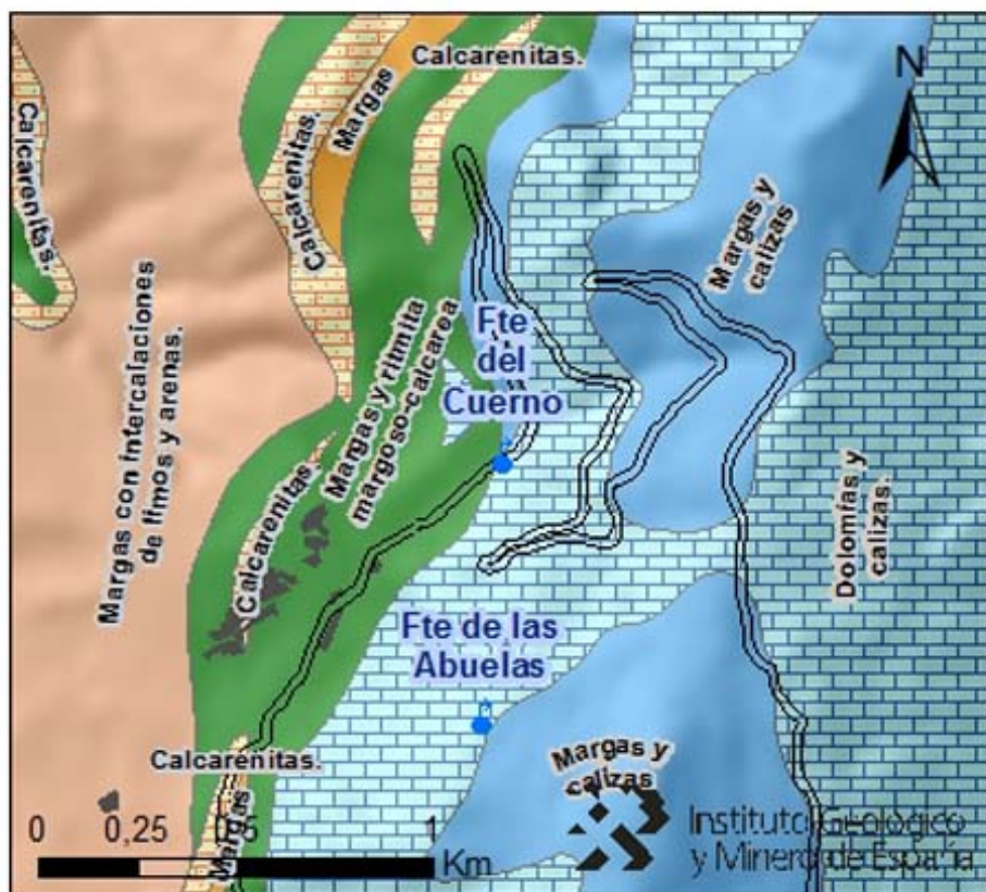
Esquema hidrogeológico (IGME Granada)
