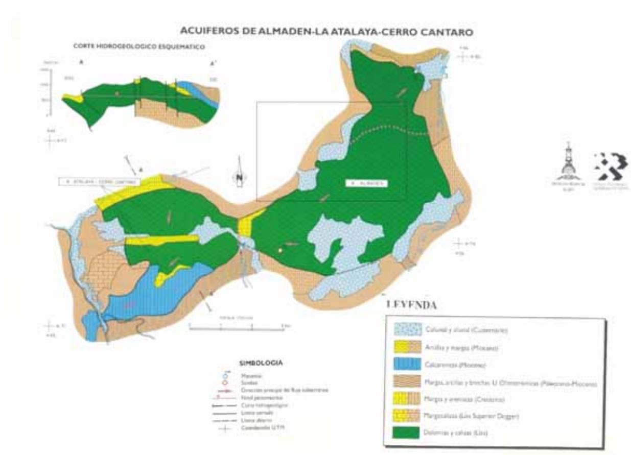
Corte y esquema hidrogeológico (IGME)
