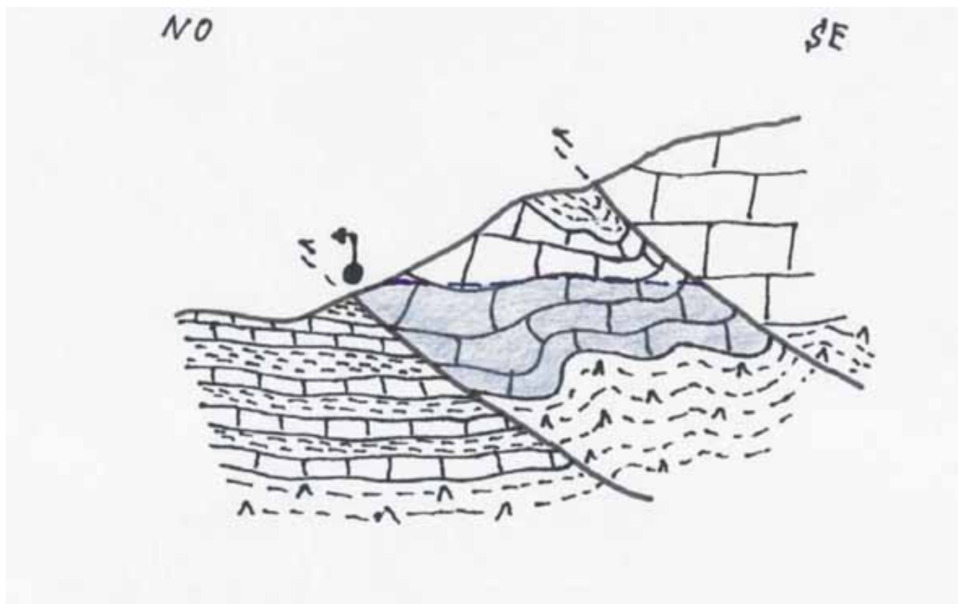
Corte hidrogeológico (IGME)
