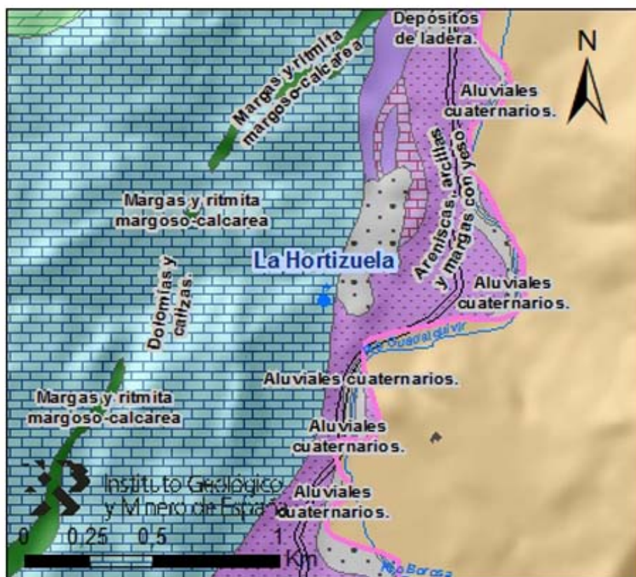
Esquema hidrogeológico (IGME Ganada)
