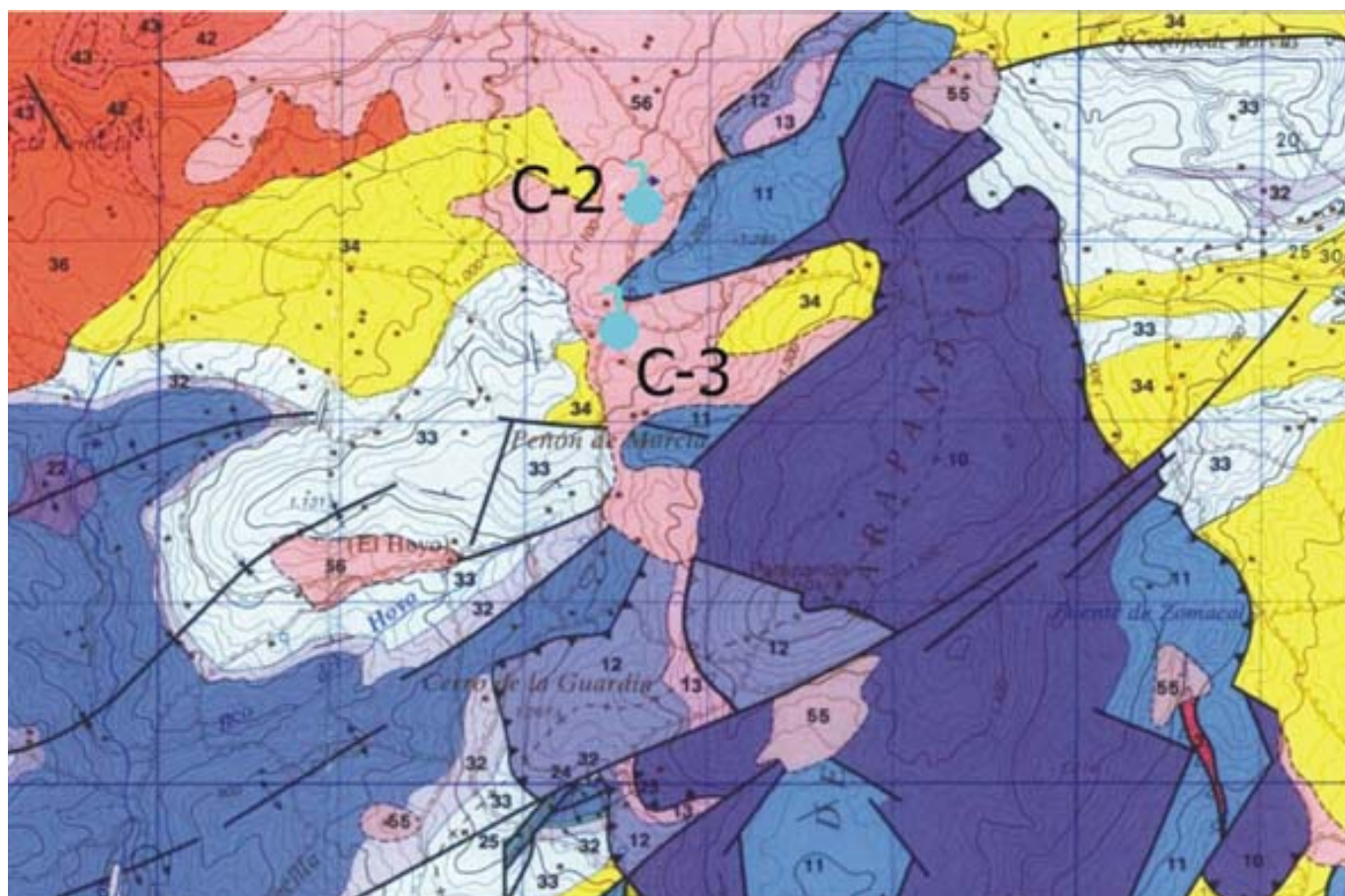
Esquema hidrogeológico (IGME Granada)
