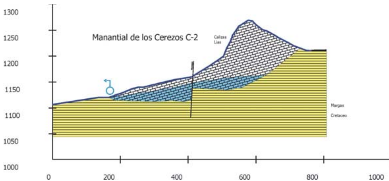
Corte hidrogeológico (IGME Granada)
