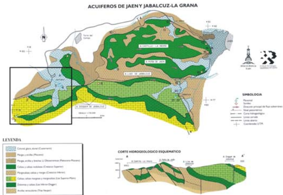
Esquema y corte hidrogeológico (IGME Ganada)
