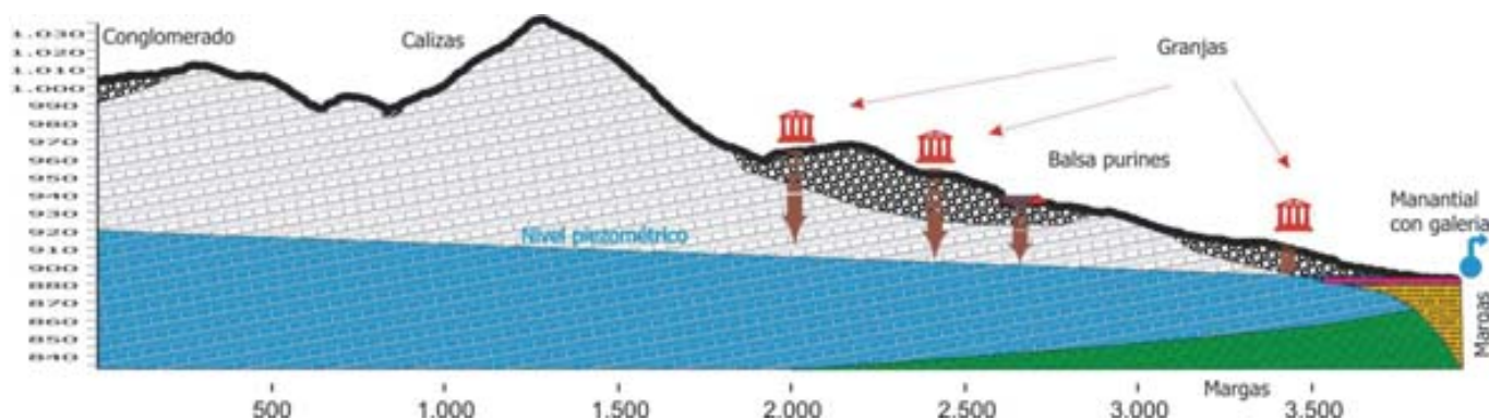
Corte hidrogeológico (IGME Granada)
