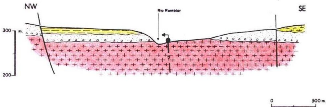
Corte hidrogeológico (IGME, Granada)
