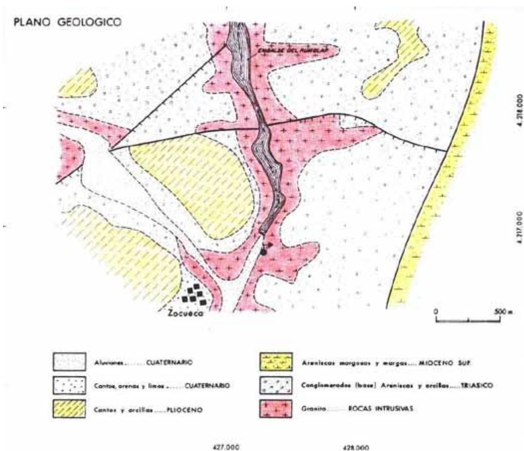
Esquema geológico (IGME Granada)
