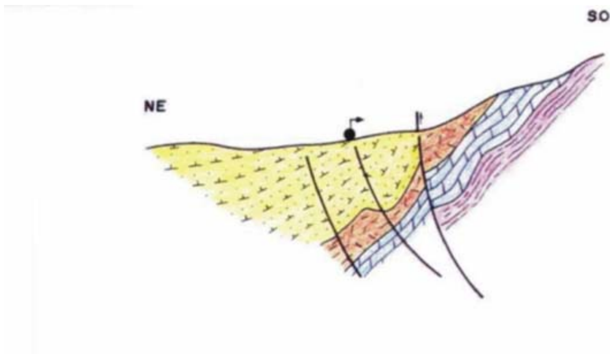
Corte hidrogeológico (IGME Granada)
