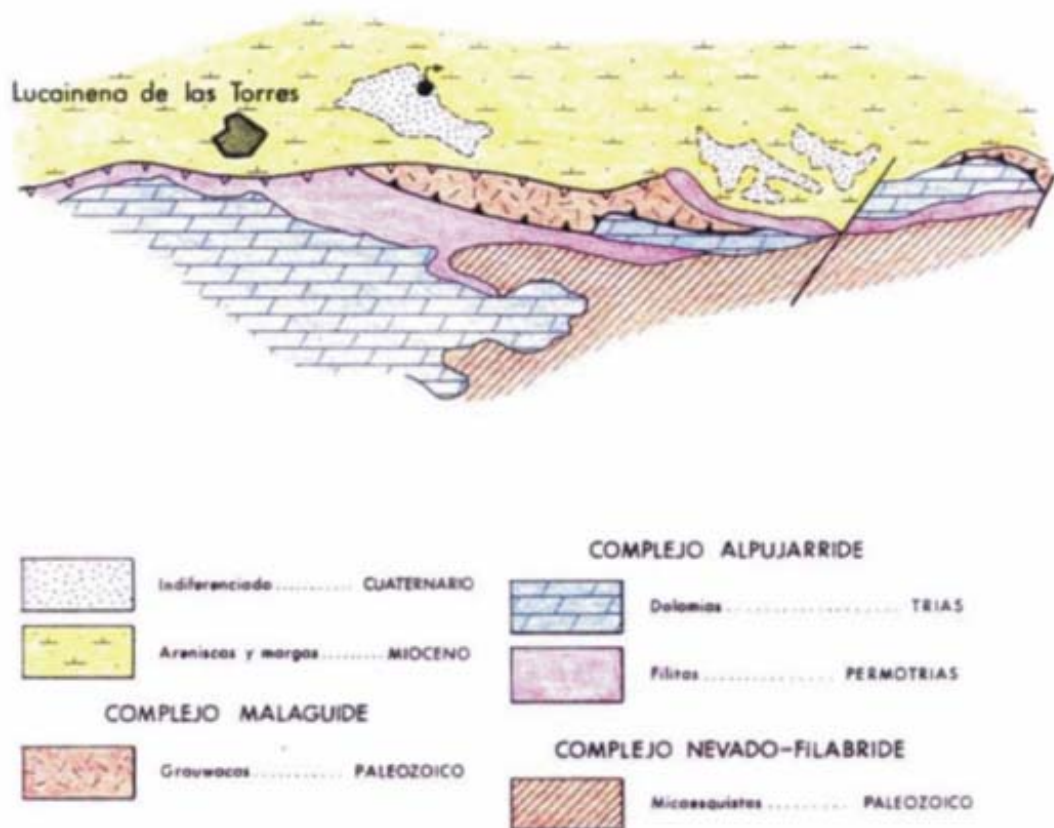
Esquema hidrogeológico (IGME Granada)
