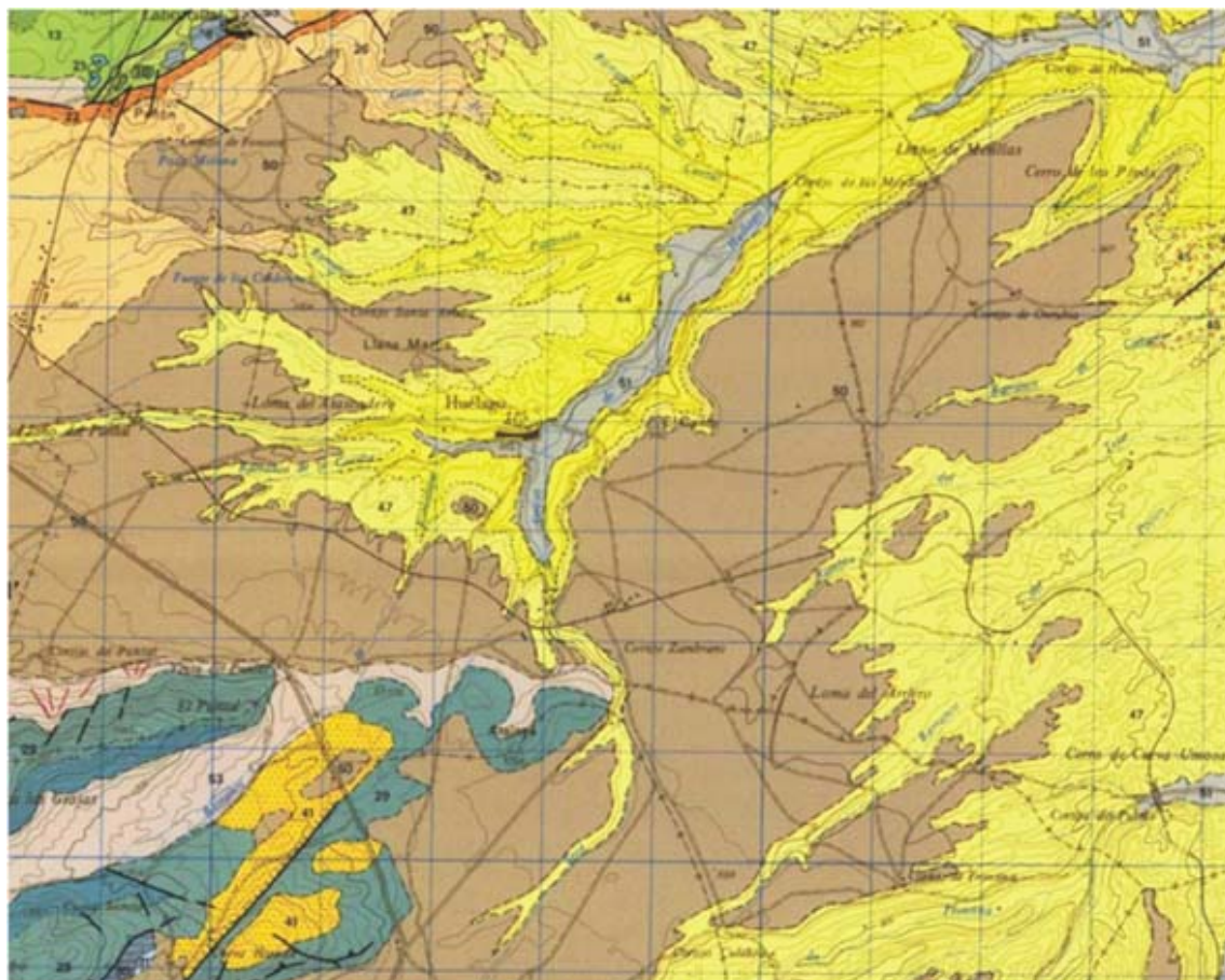
Esquema hidrogeológico (IGME Granada)
