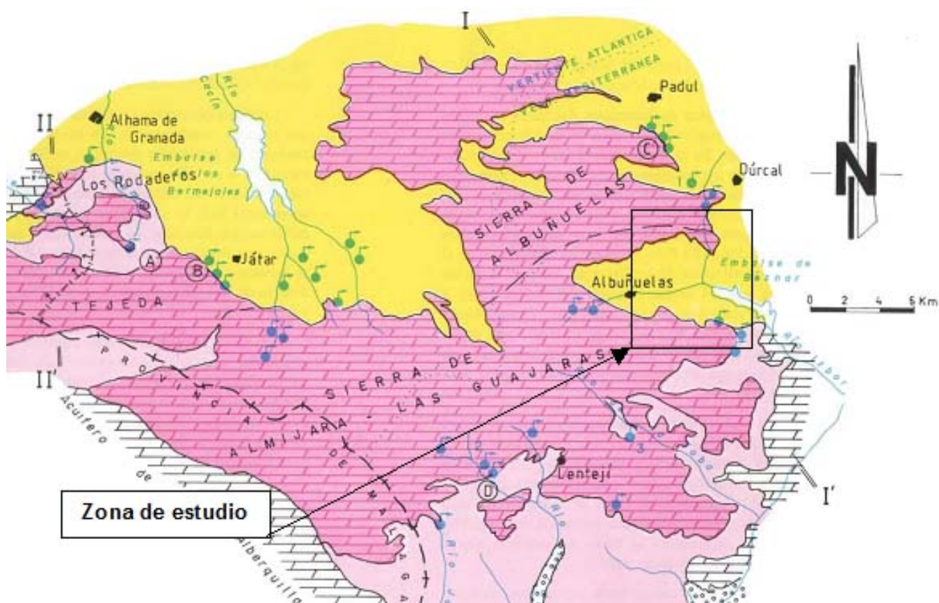
Esquema hidrogeológico (IGME Granada)
