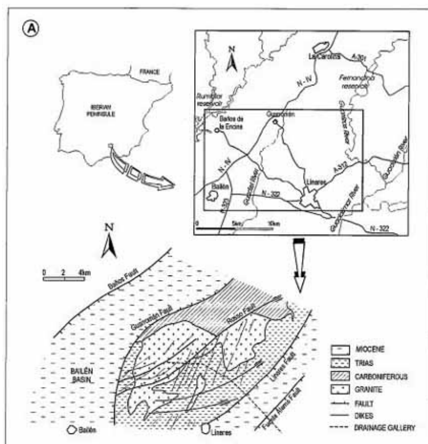
Localización del Distrito minero de Linares y mapa geológico simplificado (Geogaceta, 2002)
