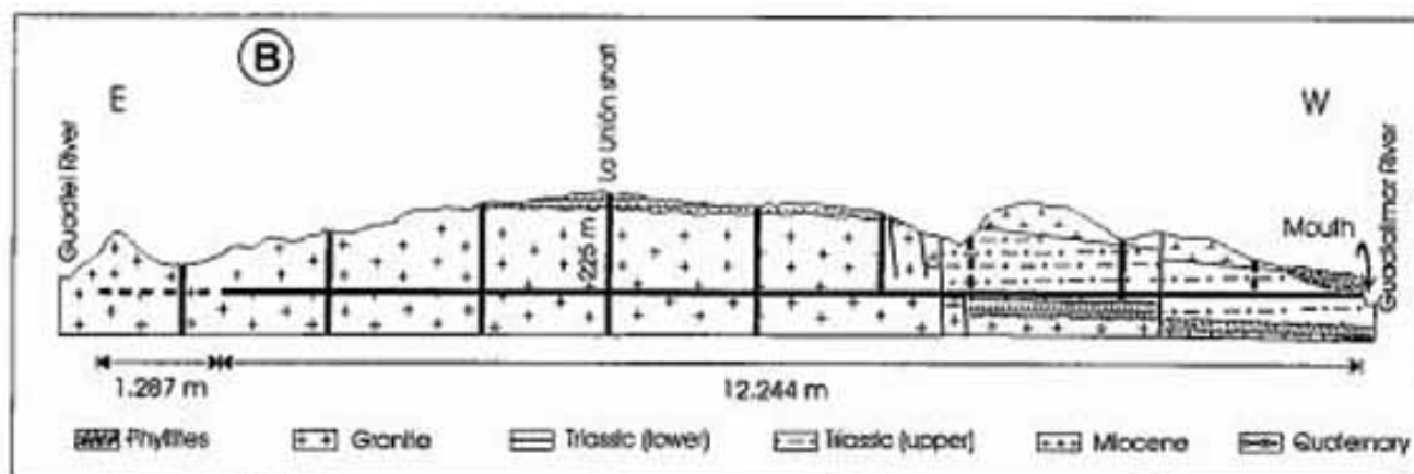
Corte geológico simplificado del Socavón minero (Geogaceta, 2002)
