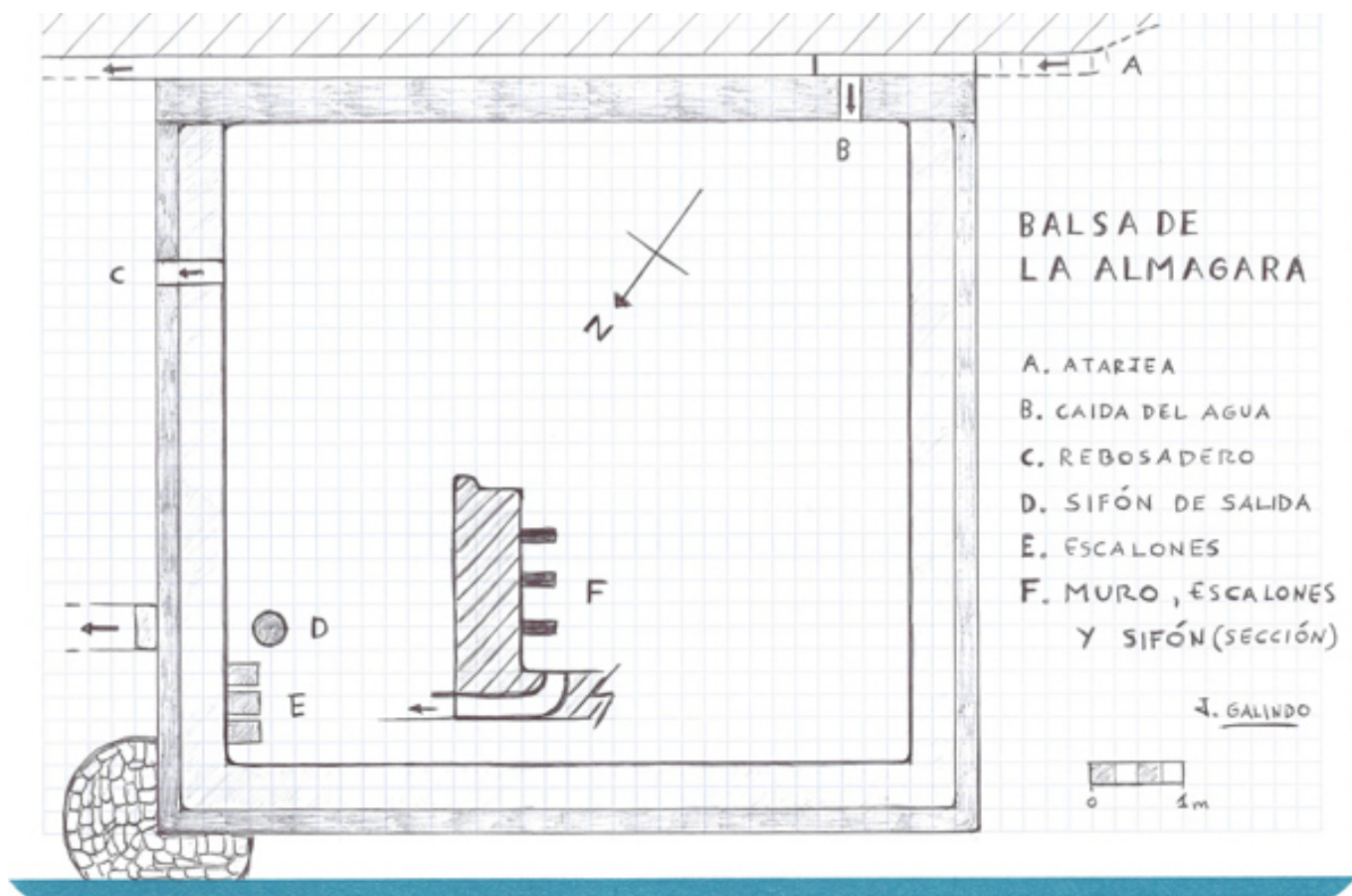
Planta y sección del muro (J. M. Galindo)
