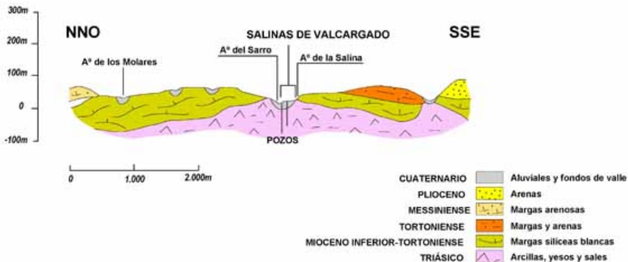
Corte hidrogeológico (Lugares de Interés Geológico de Andalucía, IGME)
