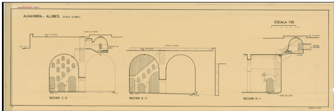
Planta y sección longitudinal. Archivo de la Alhambra (Patronato de la Alhambra)
