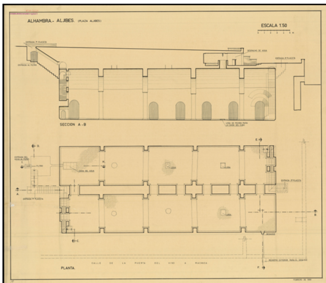
Planta y sección longitudinal. Archivo de la Alhambra (Patronato de la Alhambra)
