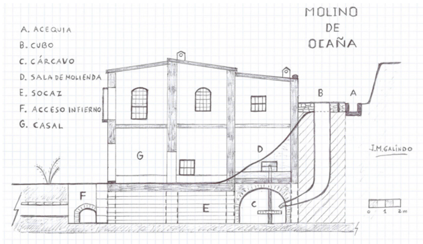
Sección transversal del Molino (J. M. Galindo López)
