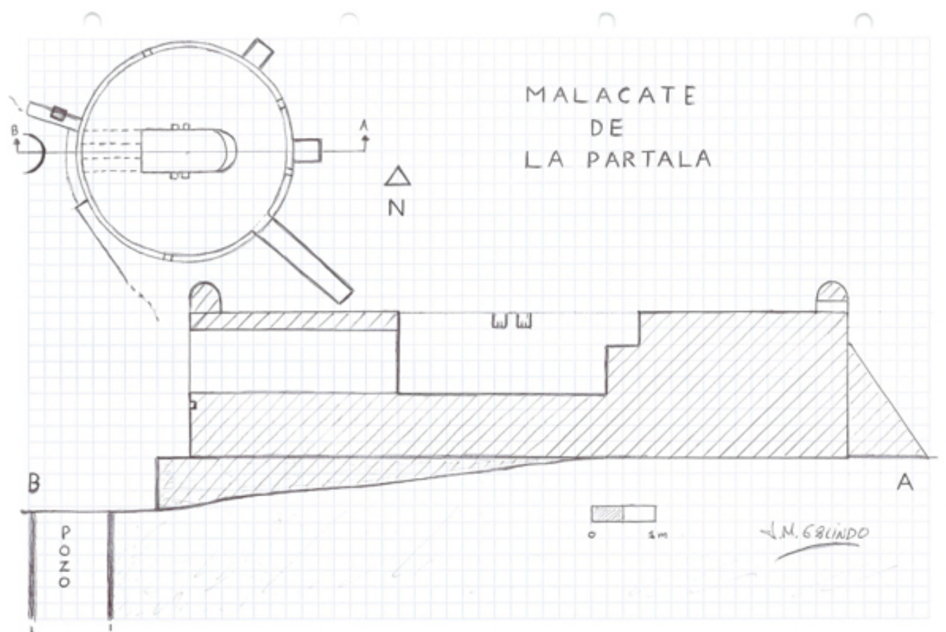
Planta y sección transversal (J. M. Galindo, febrero 2025)
