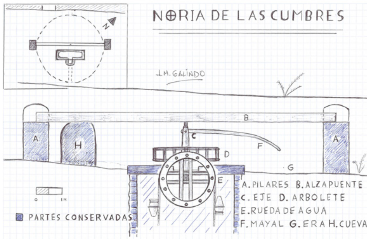
Alzado desde el sureste y esquema de funcionamiento (J. M. Galindo López, junio 2025)
