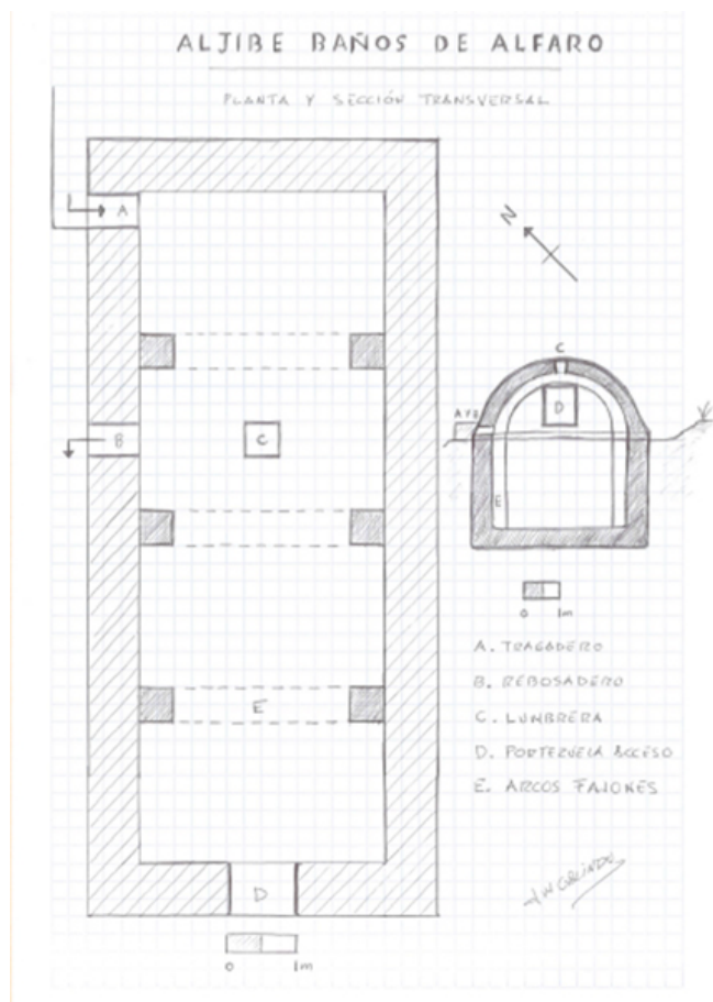
Planta y sección transversal del aljibe (J. M. Galindo López, enero 2026)
